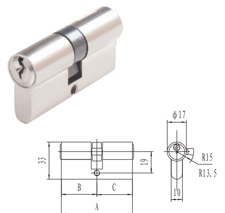
■ 标准两边钥匙锁芯 PROFILE DOUBLE CYLINDER
